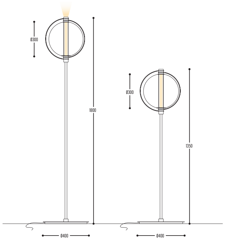
CUIABA FLOOR 180 3101-134-90454(H)-151
